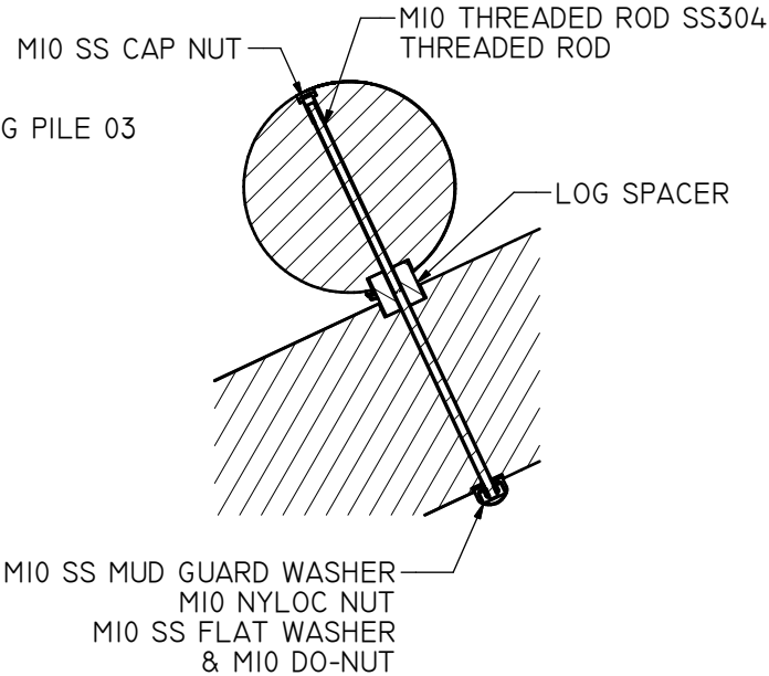
SECTION A-A ( 1 : 7 )
