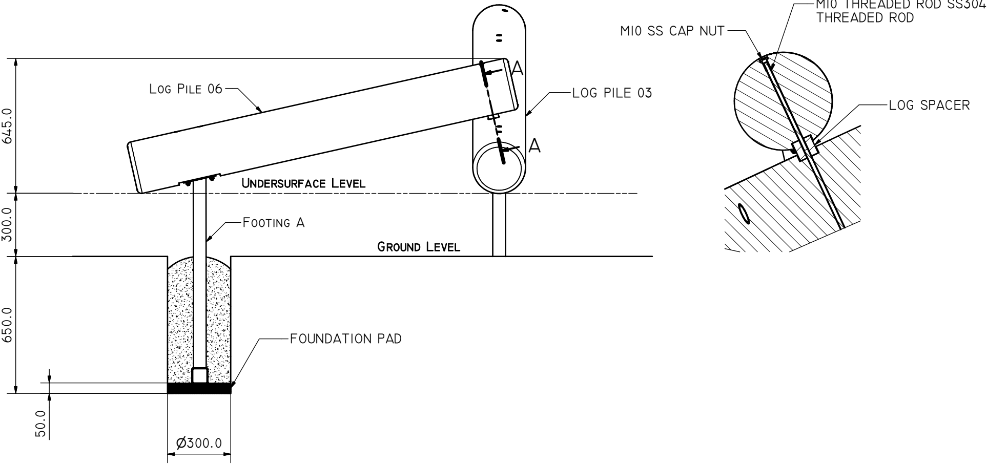
SECTION A-A ( 1 : 7 )
