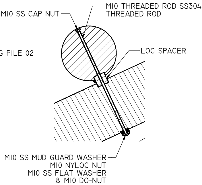
SECTION A-A ( 1 : 7 )
