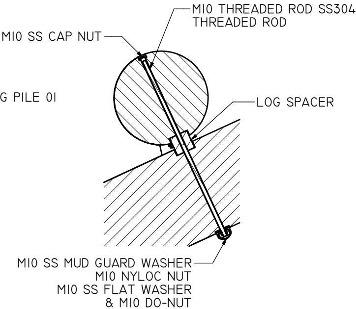
SECTION A-A ( 1:7 )
